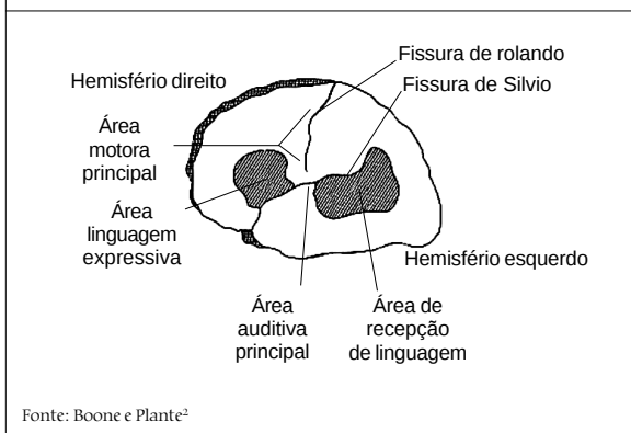
Figura 1 – Hemisférios cerebrais e principais domínios
